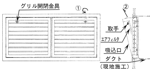
吸込Hグリル（別売品）
