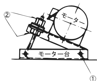
Vベルトの張り調整
