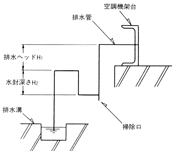
ドレン排水の施工
